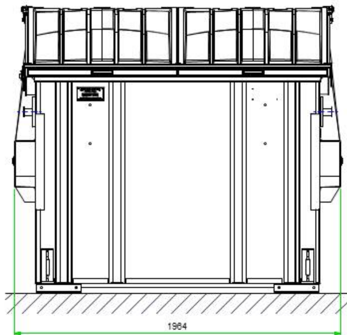
Frontlader F 7,5
